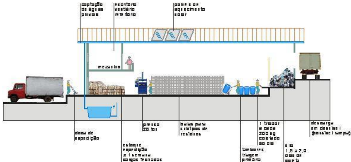
Figura 1. Sugestão de galpão de triagem em terreno em declive (MMA, 2008)
