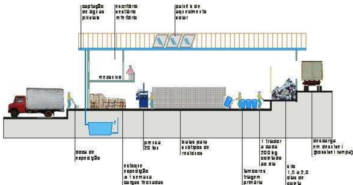
Figura 11 - Sugestão de galpão de triagem em terreno em declive (MMA, 2008).
